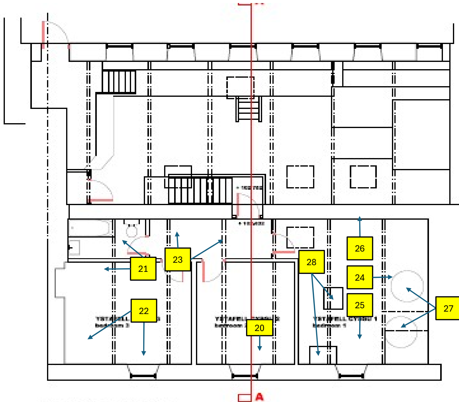
LLAWR CYNTAF first floor plan 1.100
